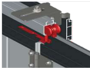
Rail de roulement en aluminium anodisé
