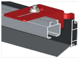
Equerre support de rail fixée sur le précadre
