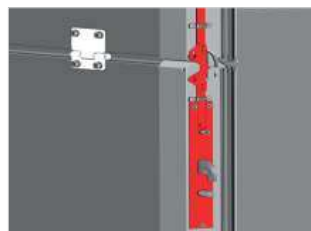
Serrure à crochets haute et basse
