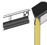
Joint haut sur traverse + joint à lèvres sur panneau haut
