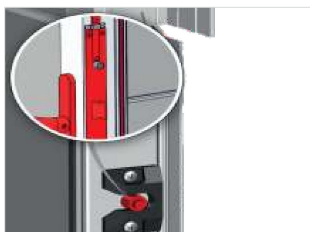
Doigts de centrage réglables par excentrique
