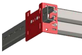
Equerre renforcée sur barre d'écartement
