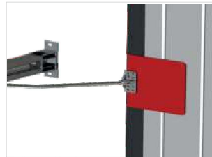
Plaque renfort pour liaison du bras moteur
