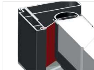
Joint à lèvres EPDM côté fermeture
