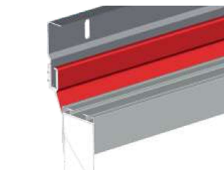
Profil support joint d'étanchéité en linteau
