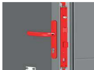
Serrure 3 points (5 points d'ancrage)
