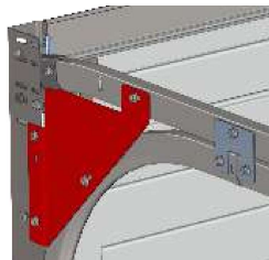
Plaque renfort sur courbes
