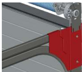
Renfort d'angle sur courbe de renvoi
