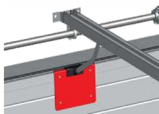
Plaque renfort pour liaison du bras moteur
