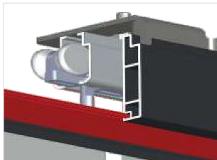
Joint d'étanchéité EPDM sur linteau
